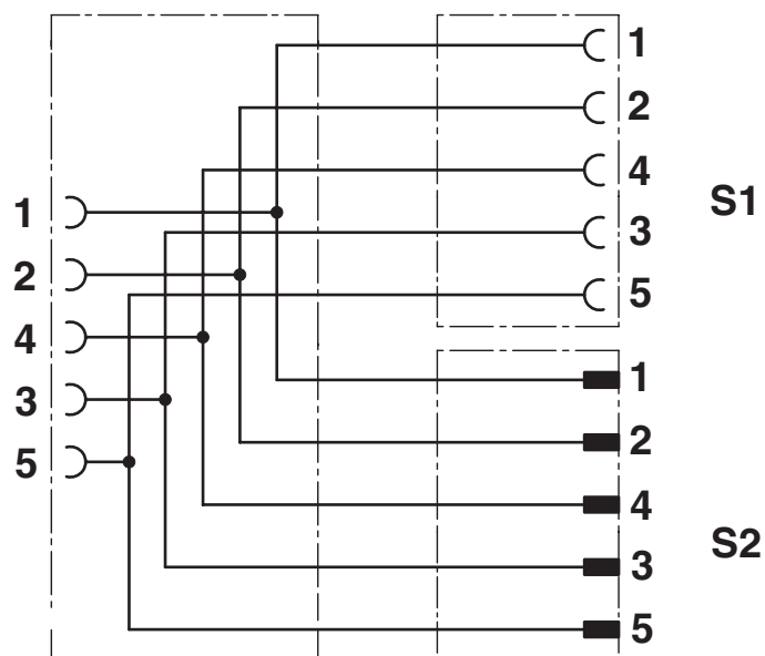
Ocupación de contactos del conector hembra M12 y del conector macho M12
