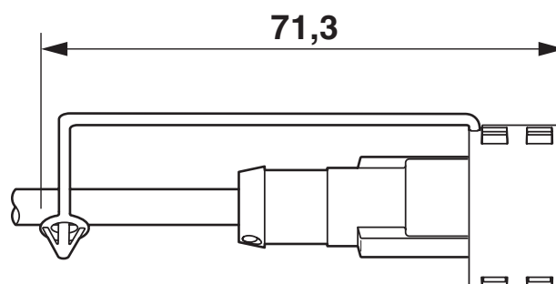
Maßzeichnung
