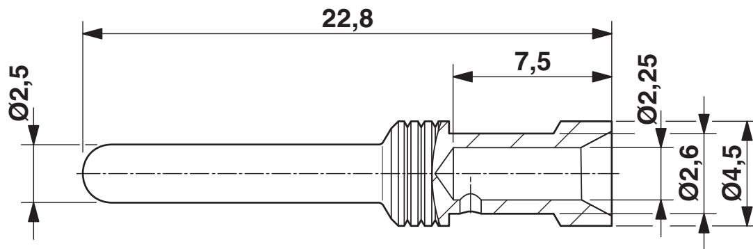
Dessin coté
