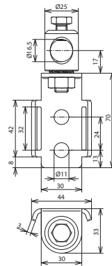
Maßbild BB SPB30 BB16 V2A AL
