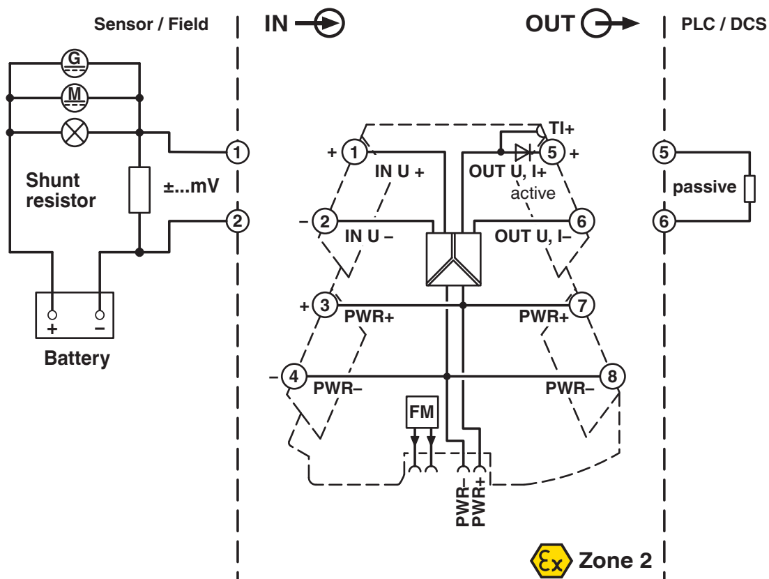
Schéma fonctionnel
