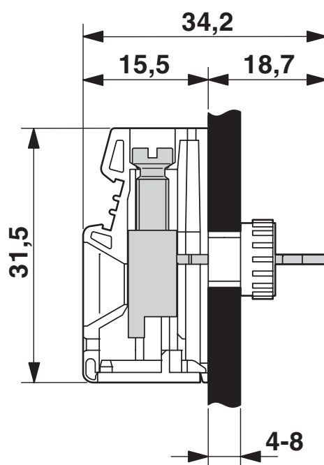
Esquema de dimensiones
