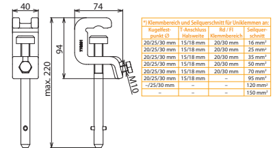
Maßbild UK K25 FL30 SQL
