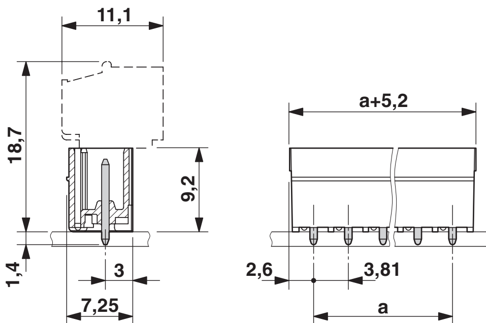
Dessin coté
