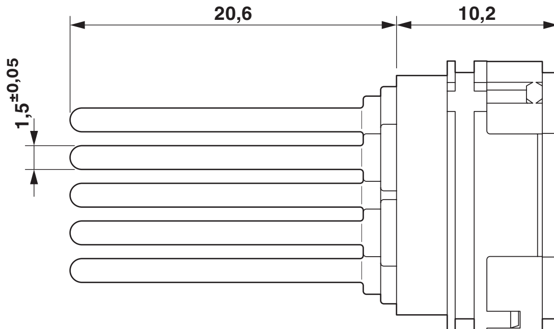
Maßzeichnung
