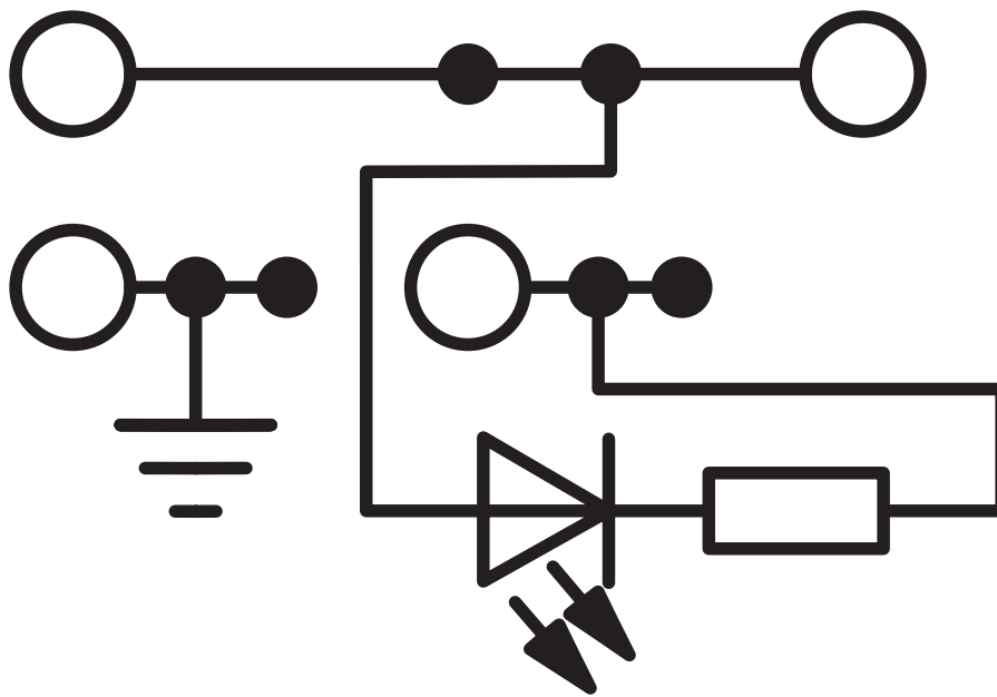
Schaltplan
