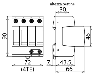
Dimensioni DG M TNS 150
