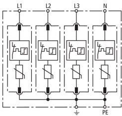
Schema di principio DG M TNS 150
