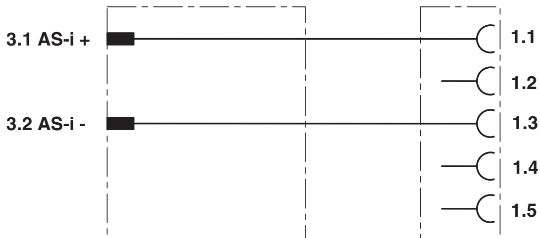
Kontaktbelegung des AS-Interface Verteilers
