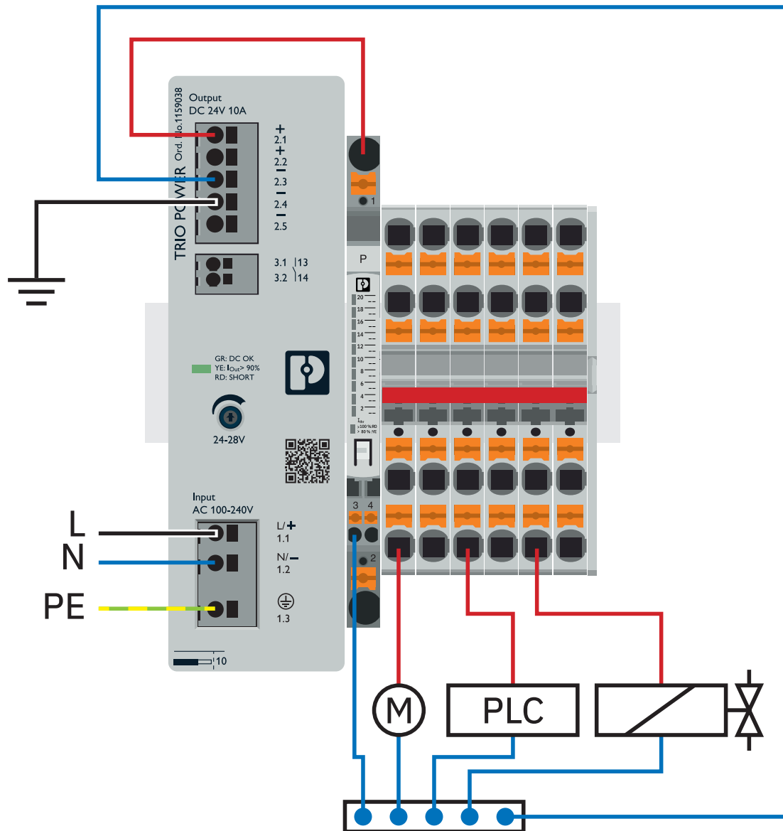
Applikationszeichnung
