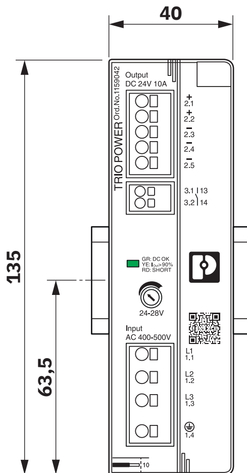
Dessin coté
