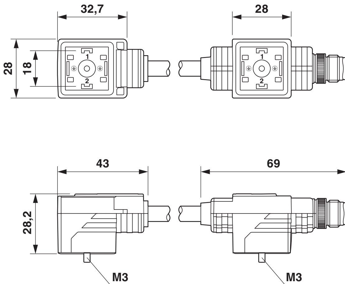
Dessin coté
