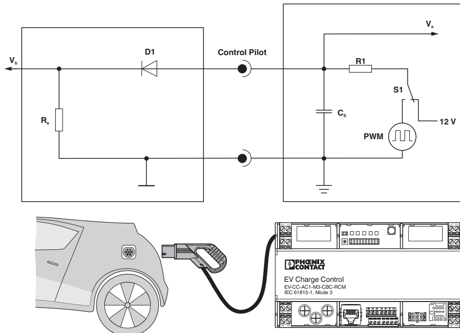
Plano esquemático
