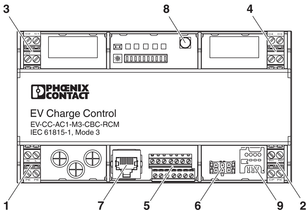
Plano esquemático
