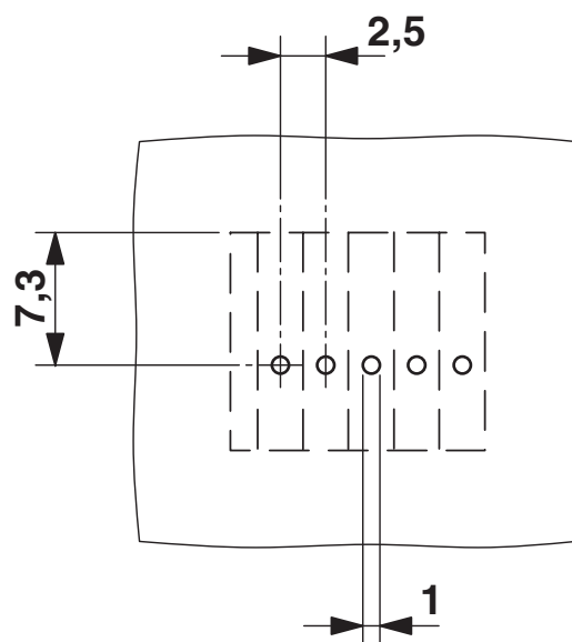
Bohrplan/Lötpadgeometrie
