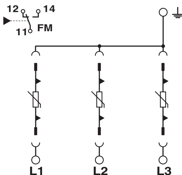
Diagrama eléctrico
