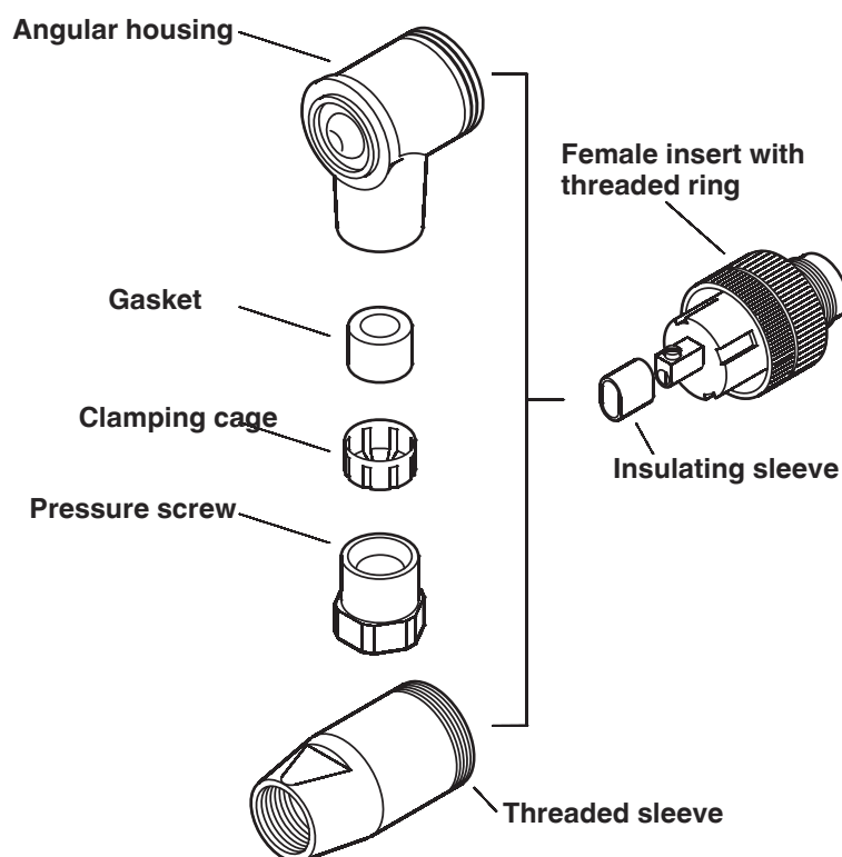
Plano esquemático
