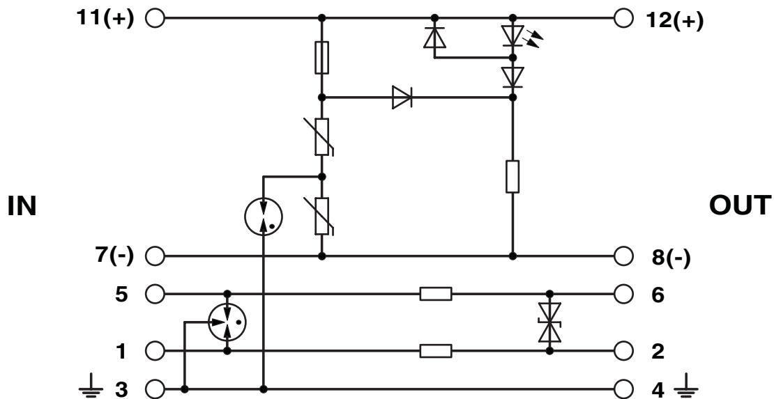
Schaltplan
