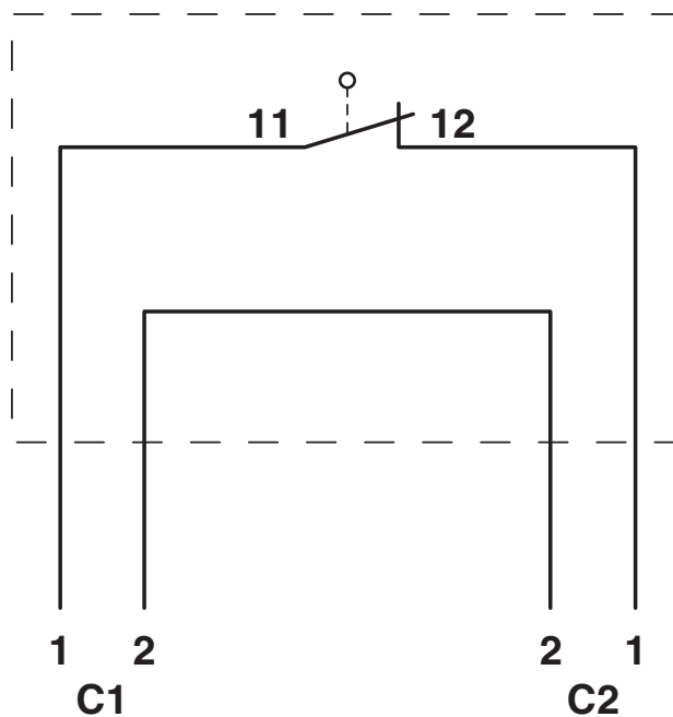
Schaltplan
