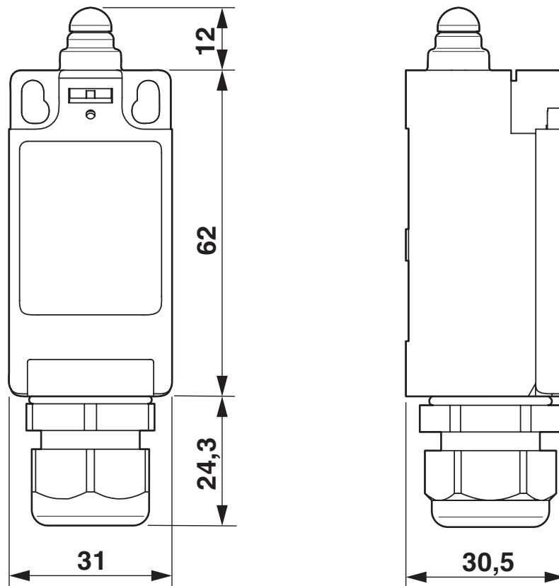
Maßzeichnung
