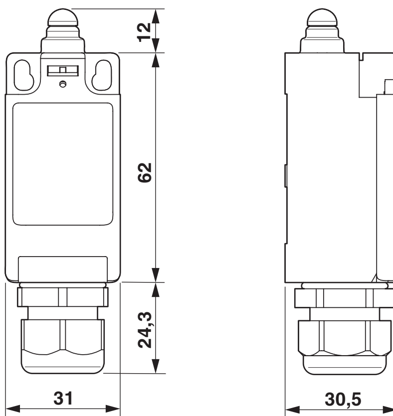
Dessin coté
