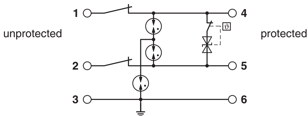
Diagrama eléctrico
