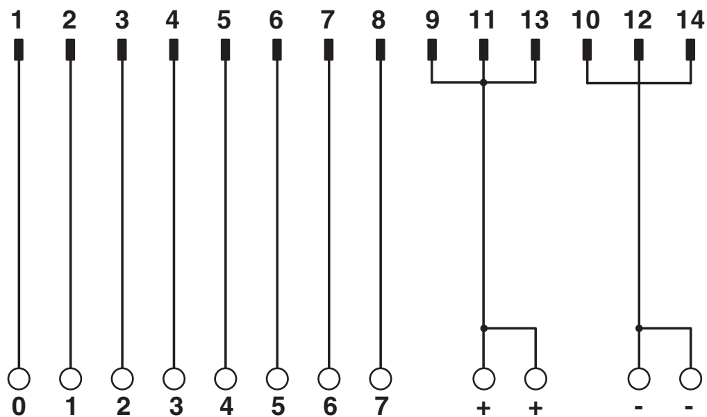
Schaltplan
