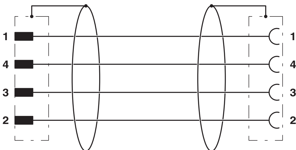
Diagrama eléctrico
