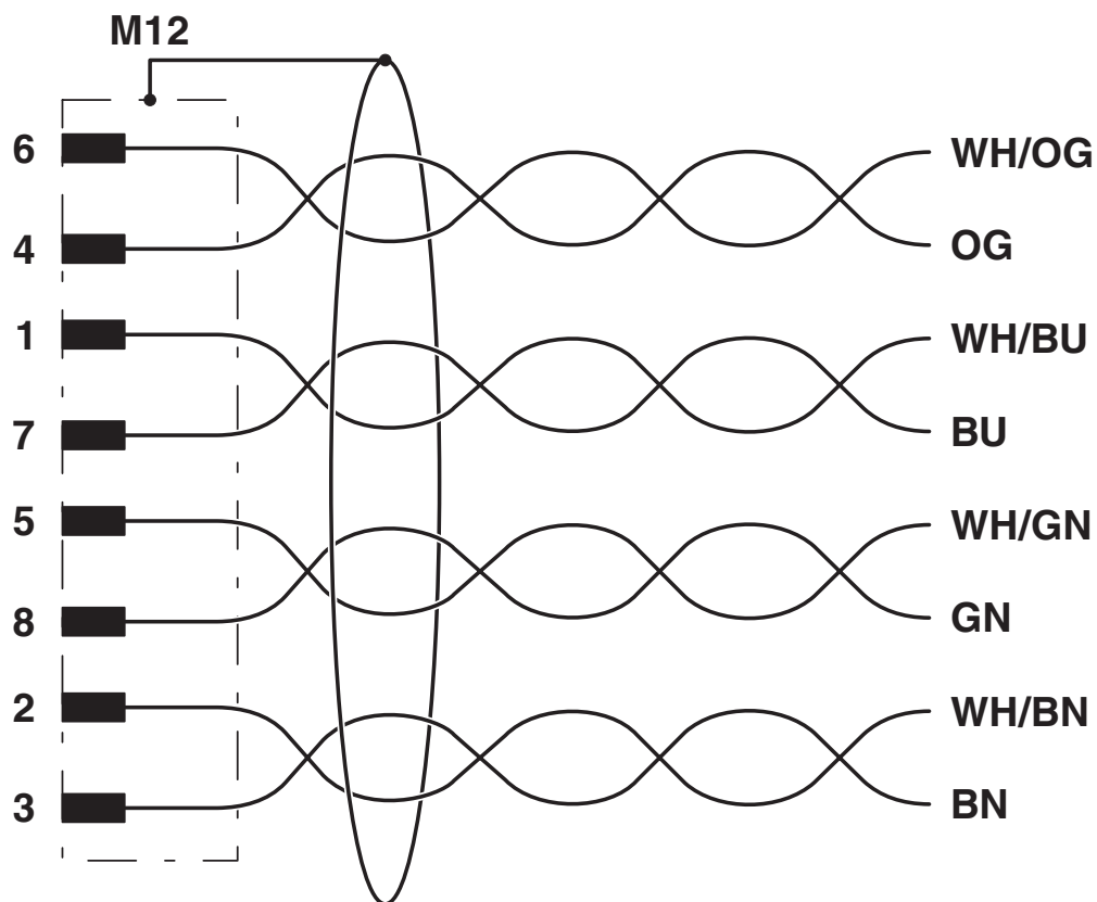
Diagrama eléctrico
