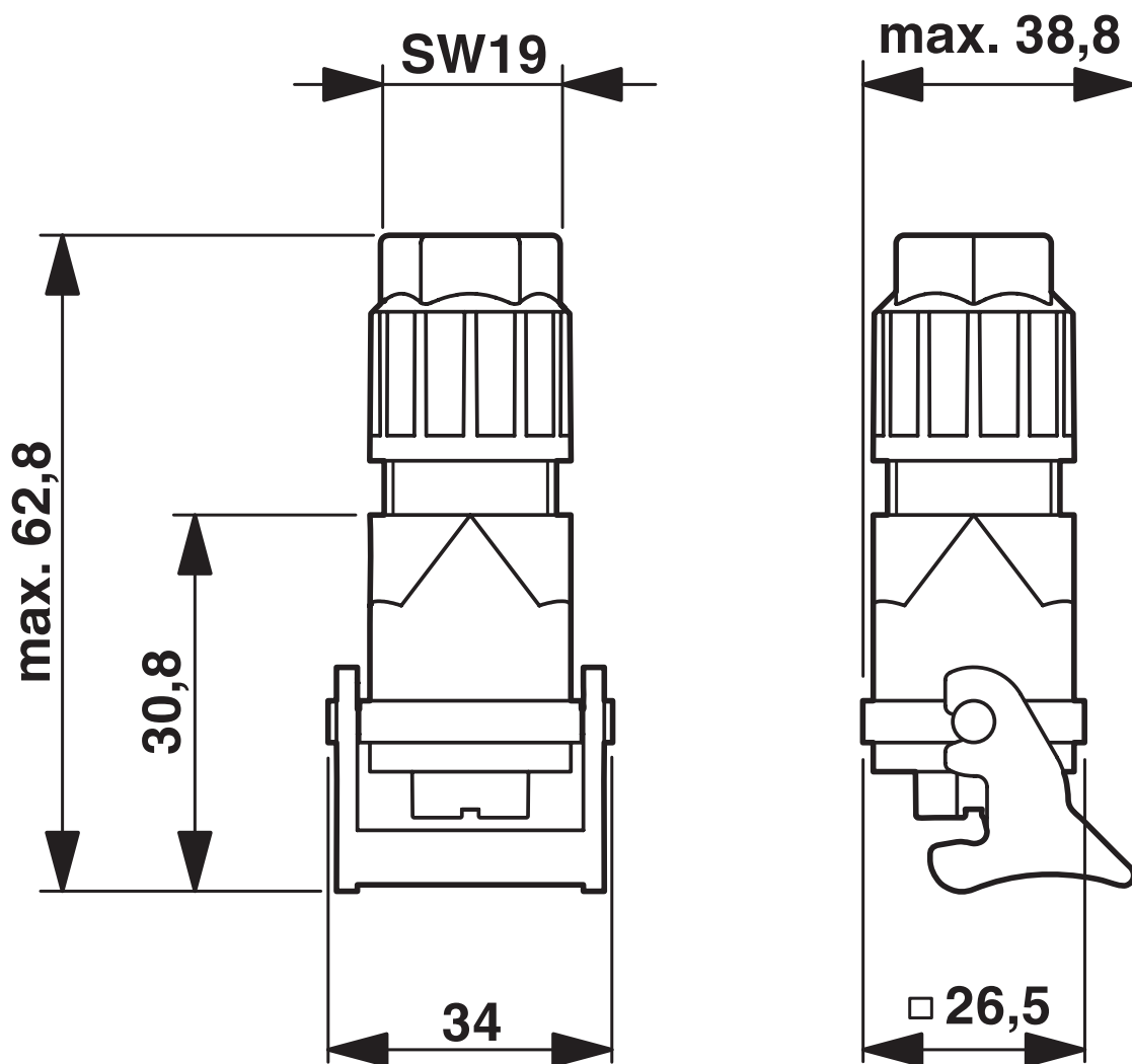
Maßzeichnung
