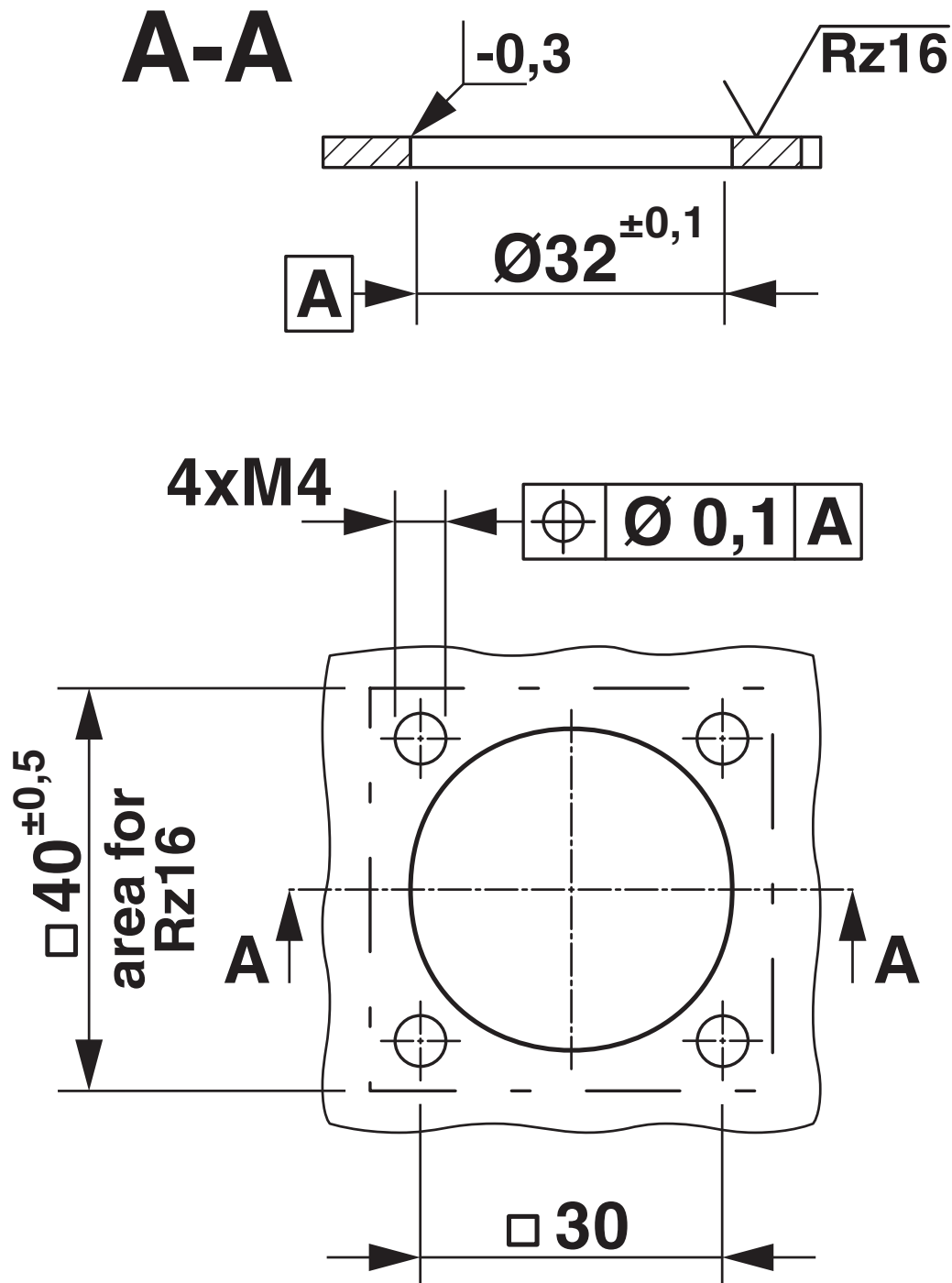
Maßzeichnung
