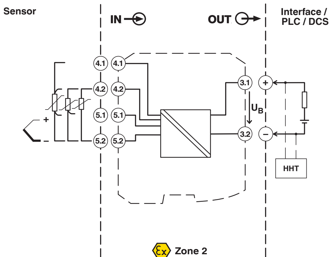
Schéma fonctionnel
