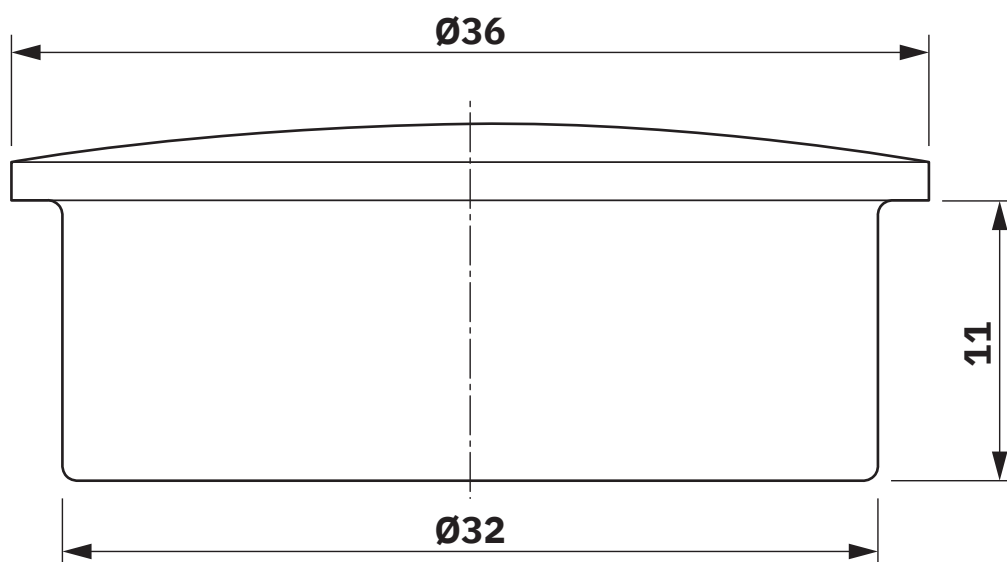
Maßzeichnung
