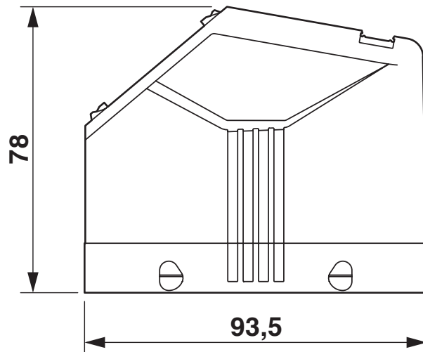
Maßzeichnung
