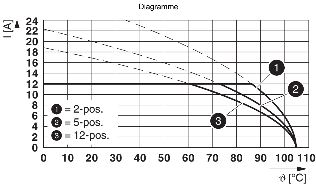
Type : ICV 2,5/...-G-5,08 avec CCV 2,5/...-G-5,08 P...THR
