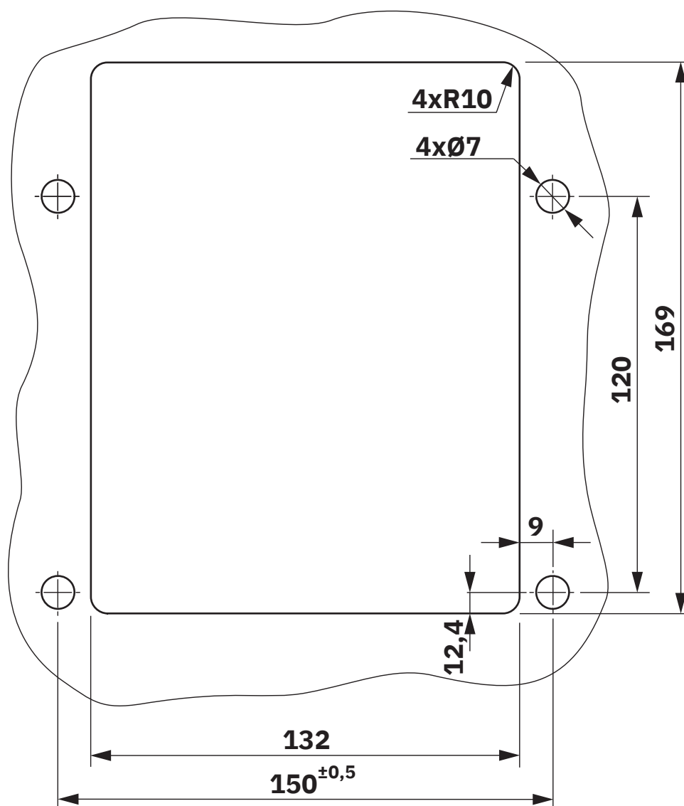
Esquema de dimensiones
