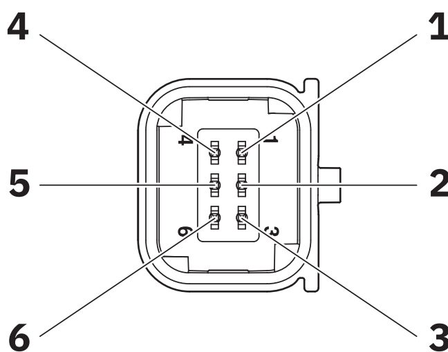
Dibujo de conexión
