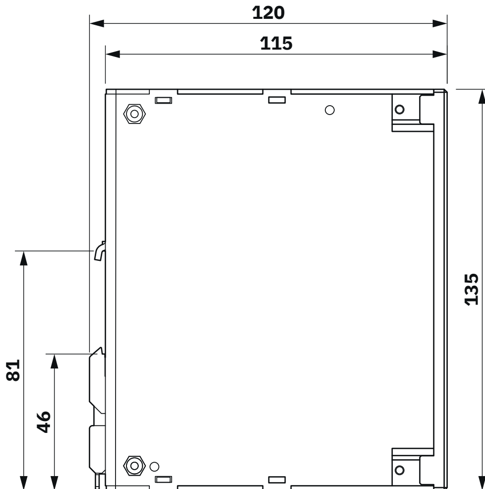
Geräteabmessungen (Maße in mm)
