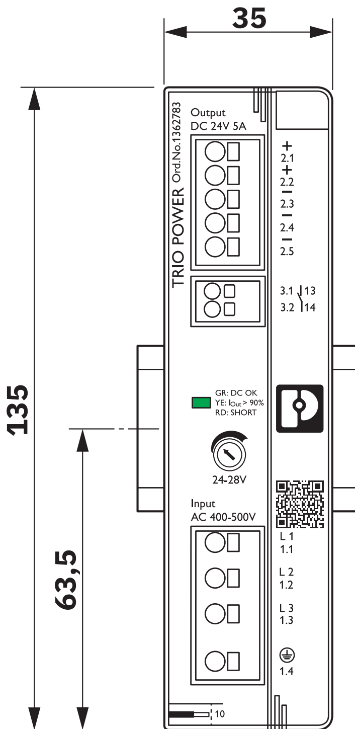
Maßzeichnung
