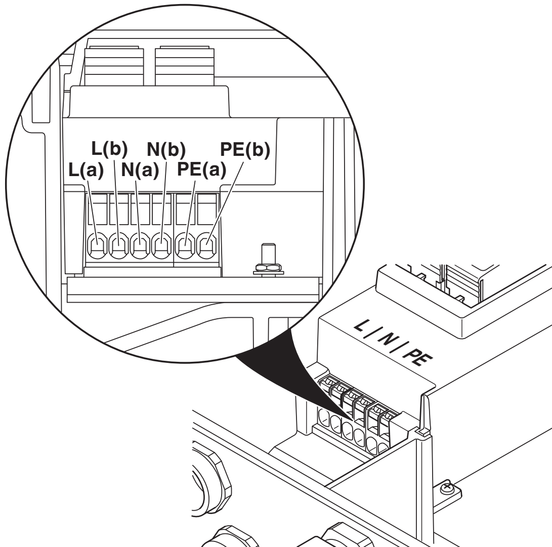
Anschlusszeichnung
