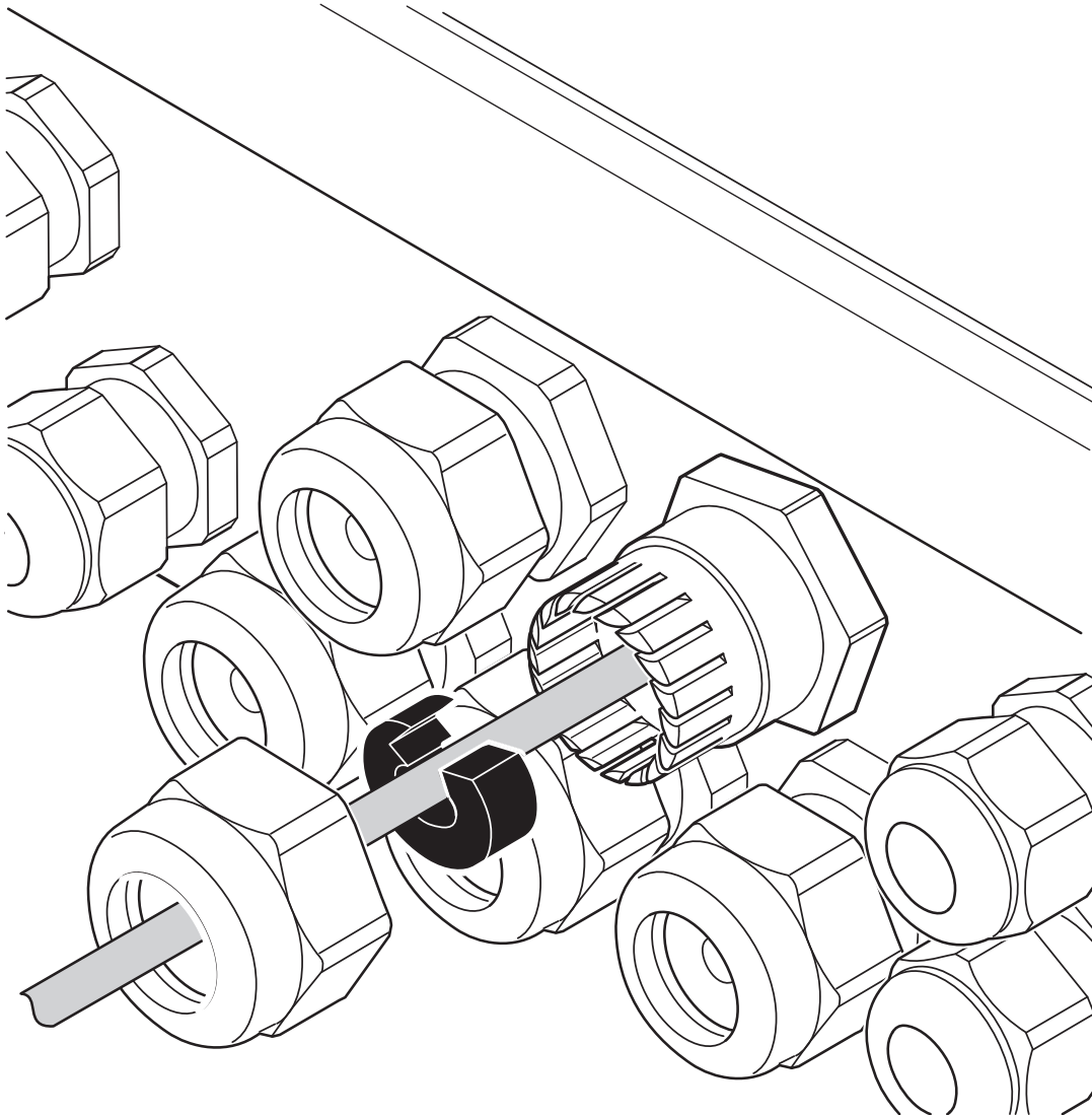
Schemazeichnung
