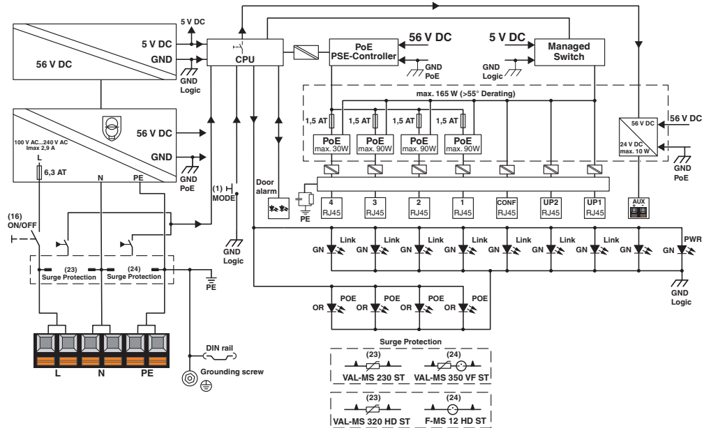
Schaltplan
