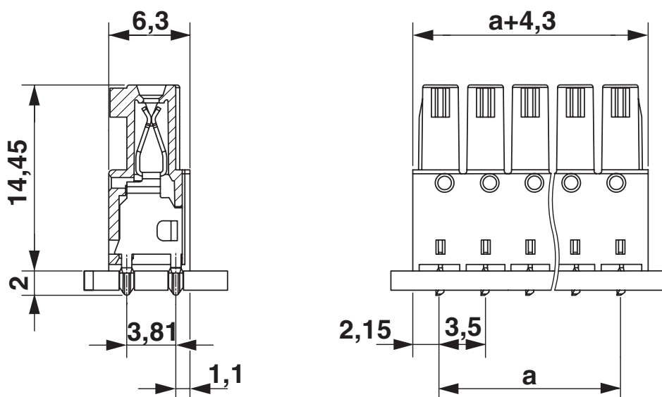
Maßzeichnung
