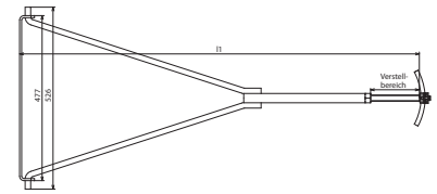
Maßbild TS 7.10 V1.45 1.75M V2A
