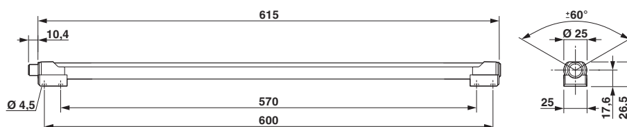
Maßzeichnung
