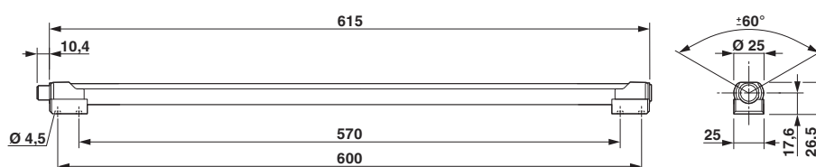
Dessin coté
