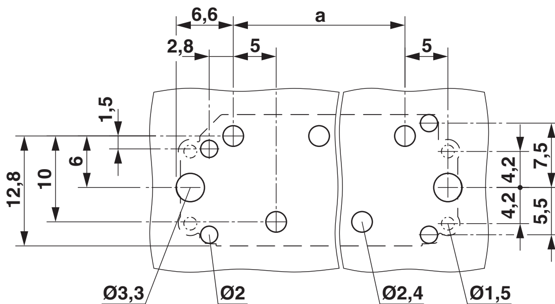
Bohrplan/Lötpadgeometrie
