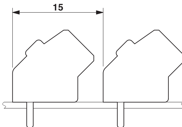
Dessin coté
