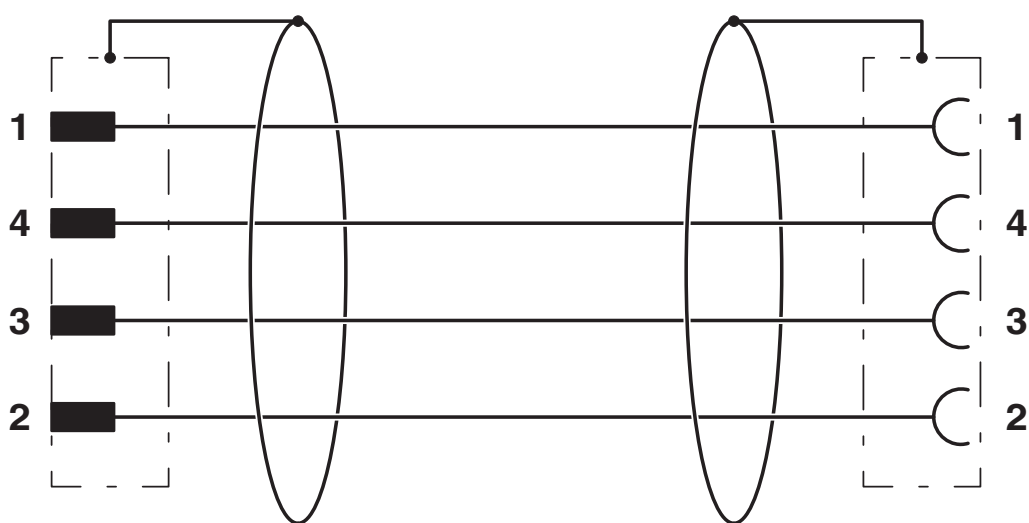
Ocupación de contactos de los conectores macho M12 / hembra M8
