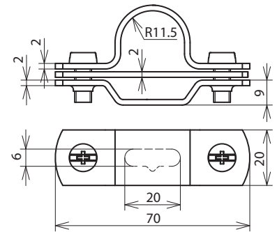
Maßbild LH ZS 23 H10 B6.5X16 V2A
