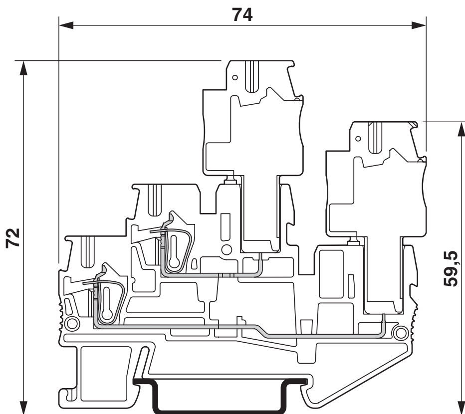
Dessin coté
