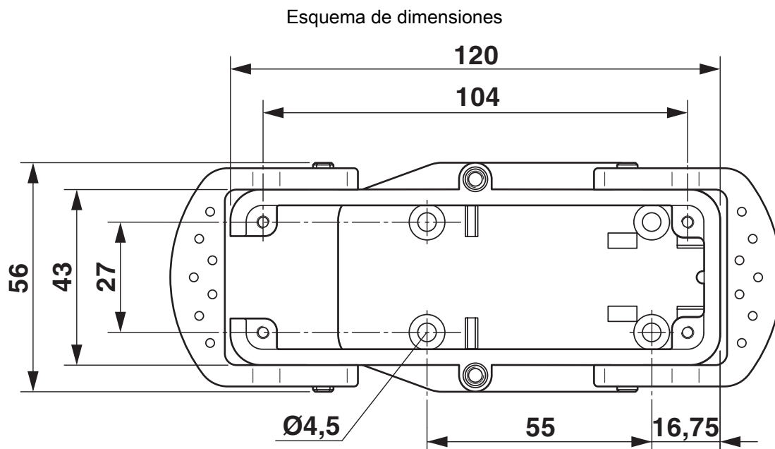
Esquema dimensiones vista desde arriba
