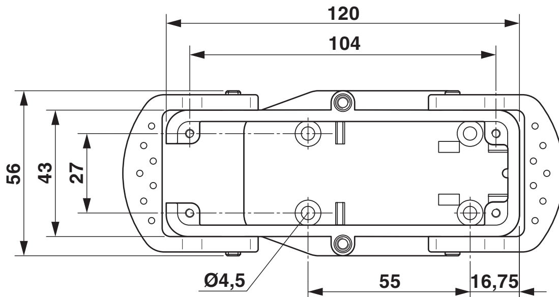
Dessin coté (vue de dessus)
