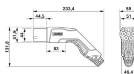
Infrastruktur-Ladestecker
