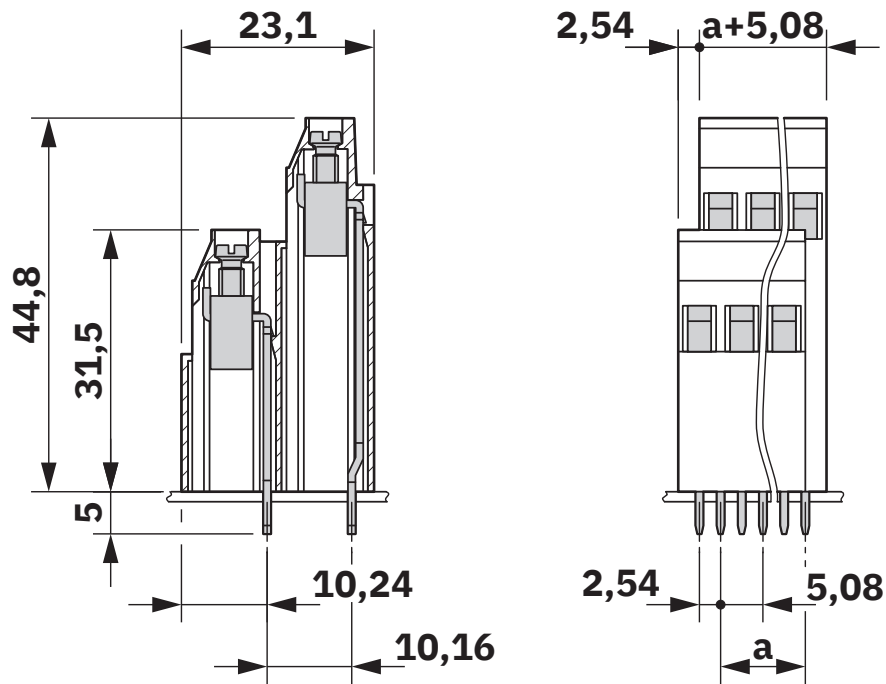
Maßzeichnung
