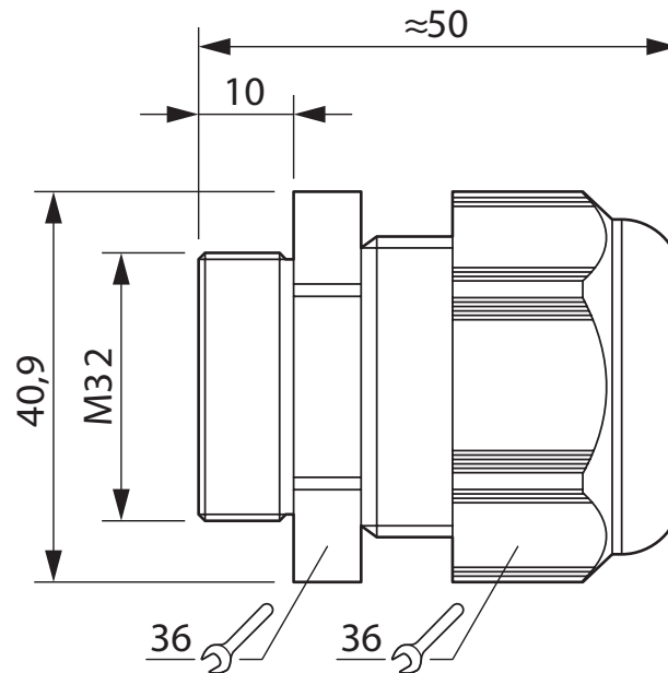
Maßzeichnung
