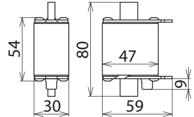
Maßbild VA NH00 280
